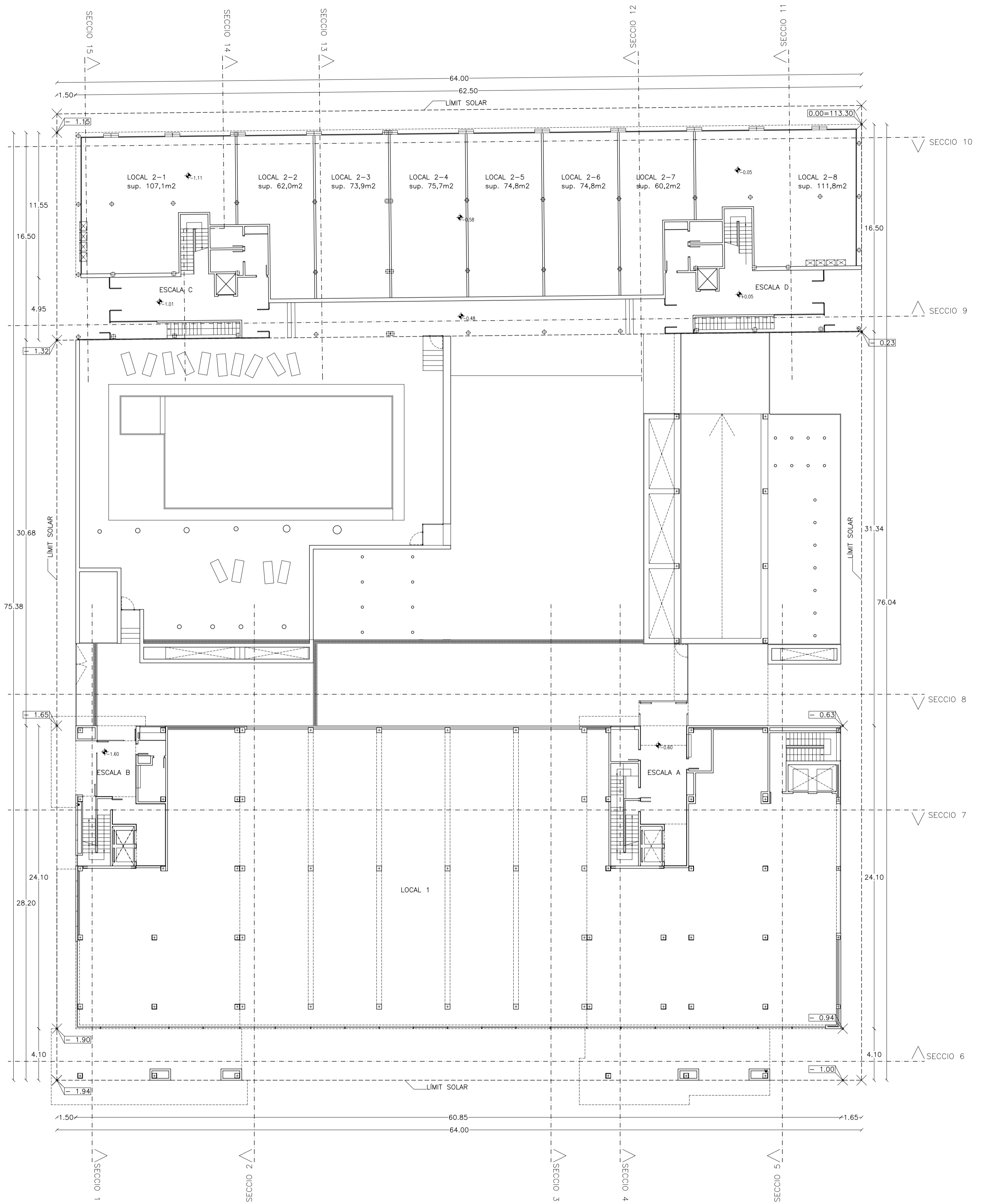
PLANTA BAIXA
